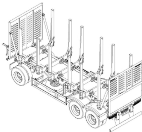
Reboque Florestal 04 Eixos para Transporte Longitudinal de Toras Reflorestadas
