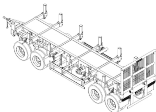
Reboque Florestal 04 Eixos para Transporte Longitudinal de Toras Nativas
