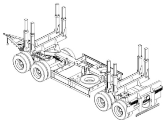
Reboque Florestal 04 Eixos para Transporte Longitudinal de Toras Nativas
