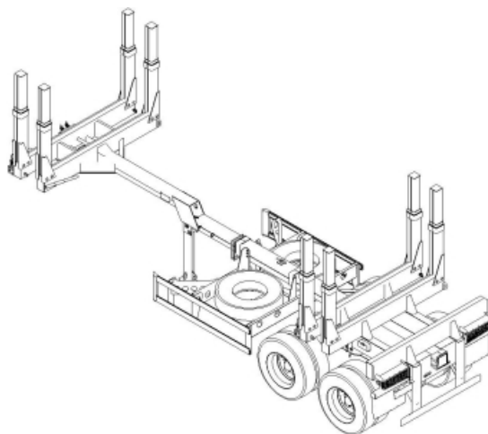
Semirreboque Alongável Florestal para Transporte Longitudinal de Toras Nativas
